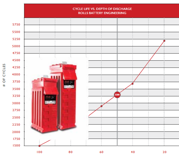
4 KS 25P
